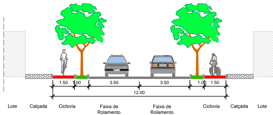
PERFIL AA TIPOLOGIA 5 ESC. 1/150
