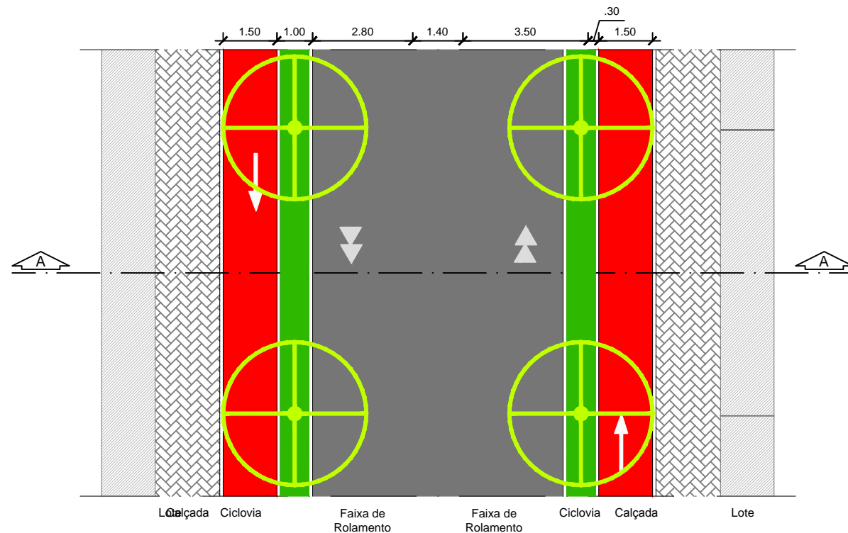
PLANTA TIPOLOGIA 5 ESC. 1/150
